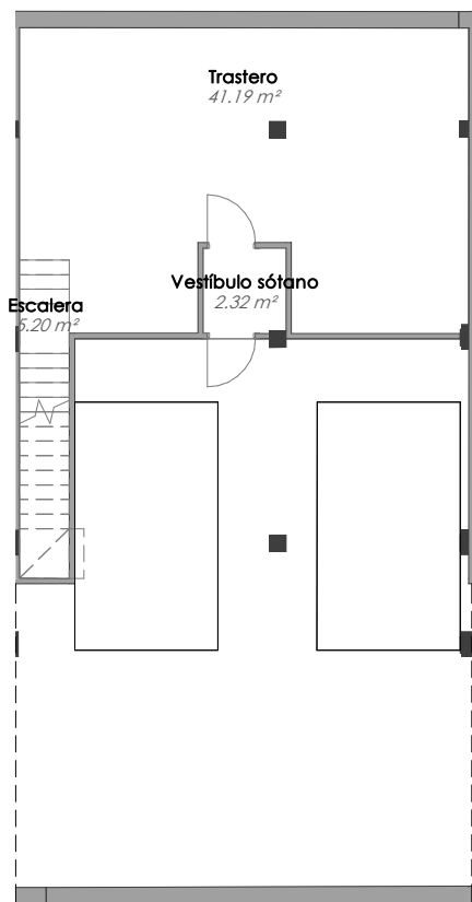
PLANTA SÓTANO
