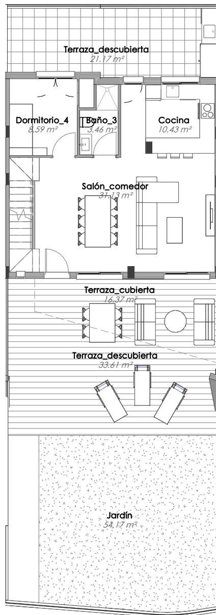
PLANTA 0
