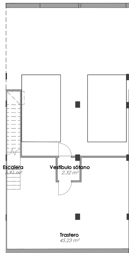
PLANTA SÓTANO
